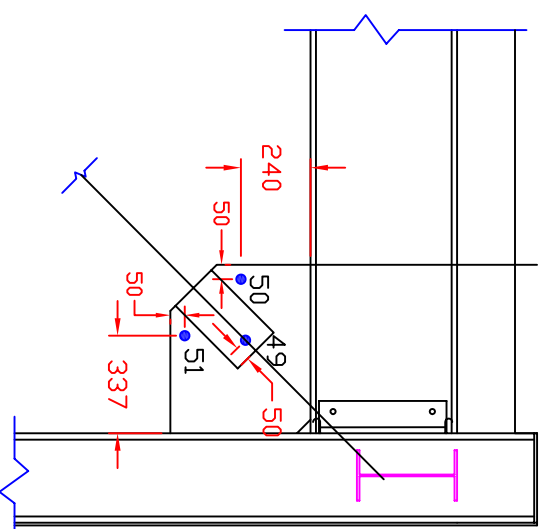
UPPER GUSSET PLATE, TYP.
